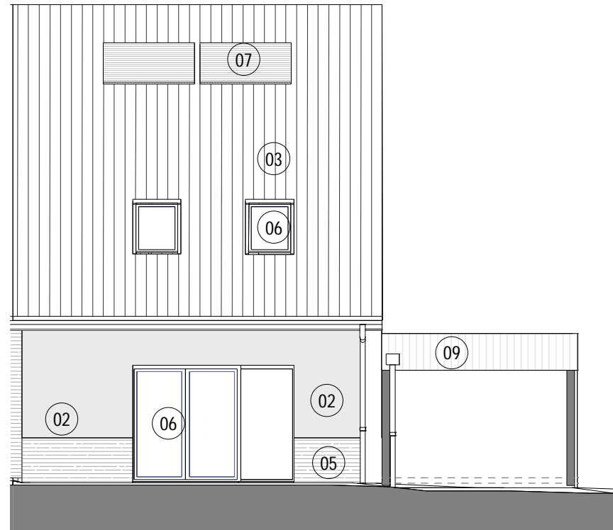
1 ML9A Maison 14 ELEVATION EST
