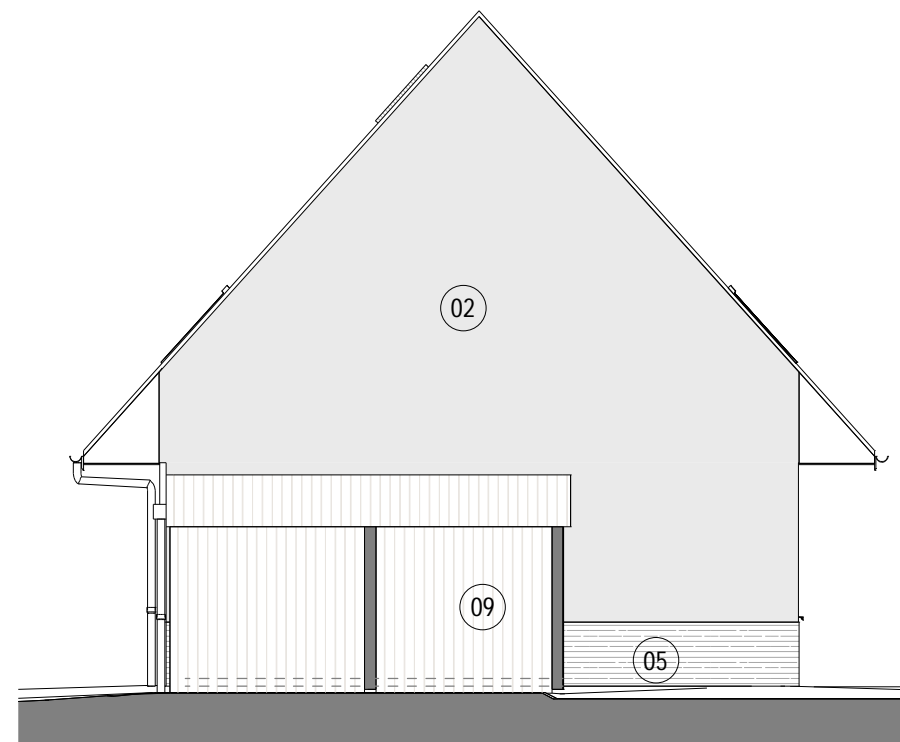
3 ML9A Maison 14 ELEVATION NORD
