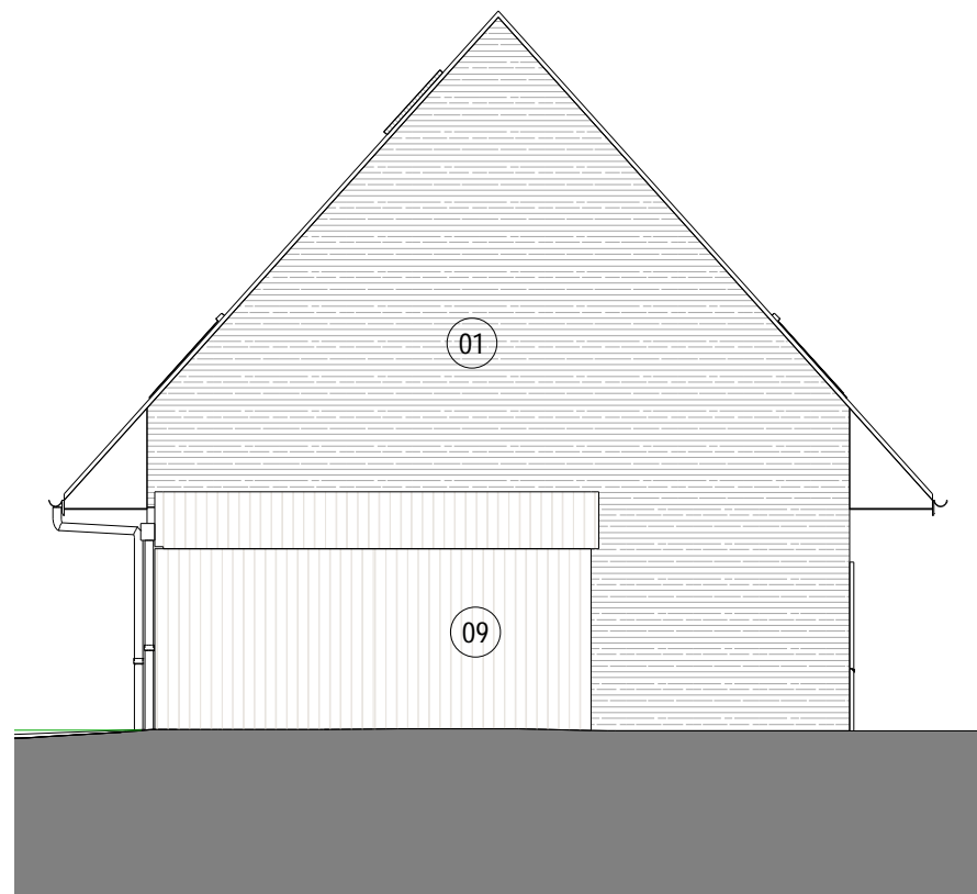
3 ML10 Maison 16 ELEVATION OUEST
