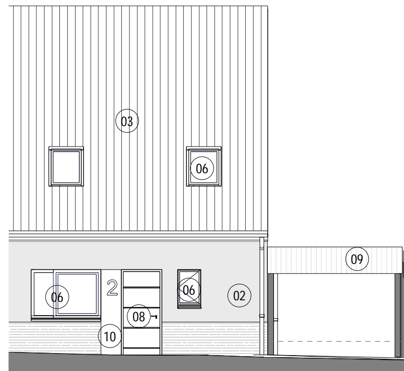
1 ML10 Maison 17 ELEVATION SUD
