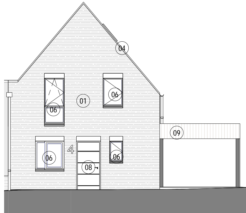
1 ML4 Maison 03 ELEVATION NORD OUEST
