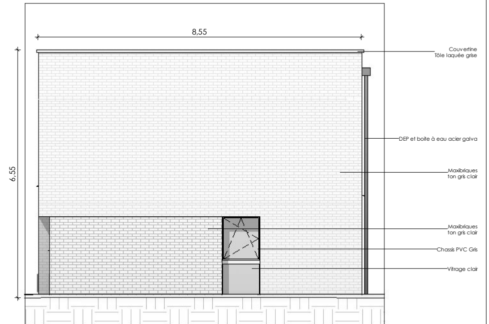
Façade latérale - Nord/Est
