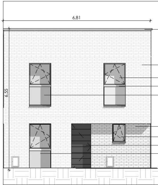
Façade avant - Nord/Ouest
