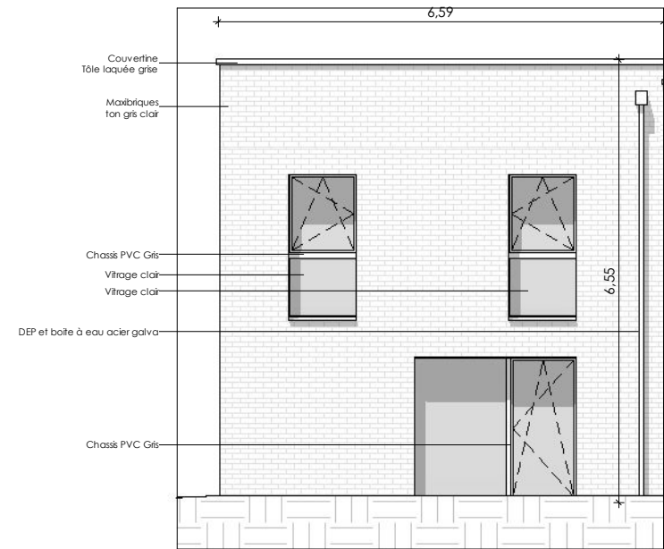
Façade arrière - Sud/Est
