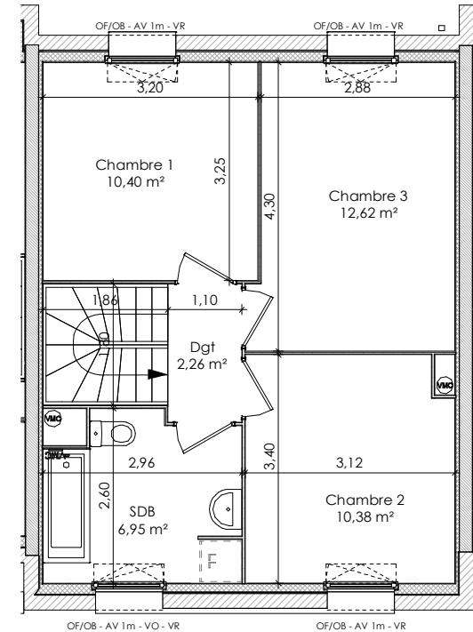
Etage SH = 42,61 m 2
