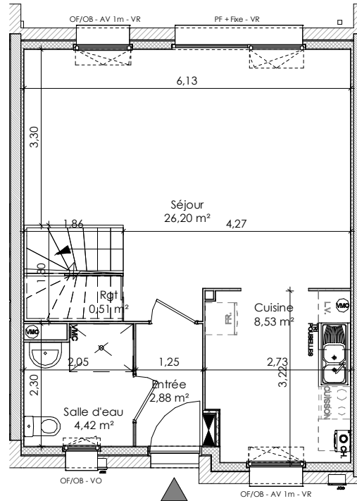
Rez-de-chaussée SH = 42,54 m 2
