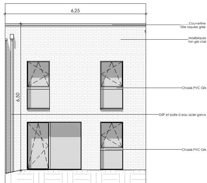
Façade arrière - Sud/Est
