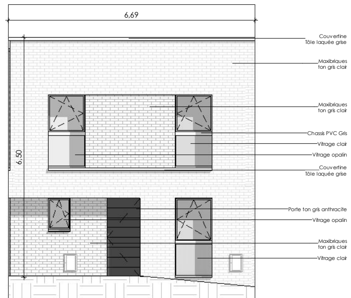
Façade avant - Nord/Ouest
